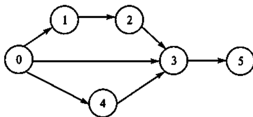
Рис. 2.20. Диаграмма последовательности работ при строительстве здания
