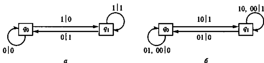
Рис. 7.4. Графы элементов памяти:
