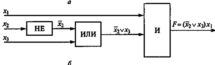
Рис. 4.8. Логические схемы булевой функции F :
