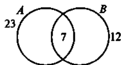
Рис. 1.21. Схематическое изображение условия задачи 15
