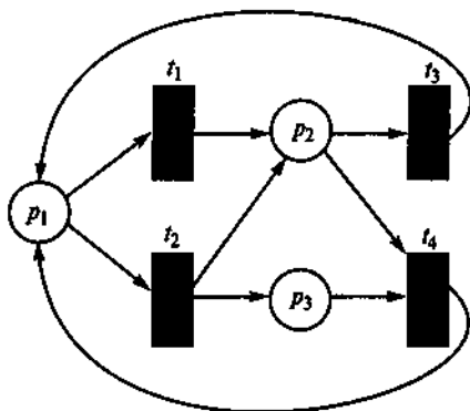
Рис. 2.22. Сеть Петри
