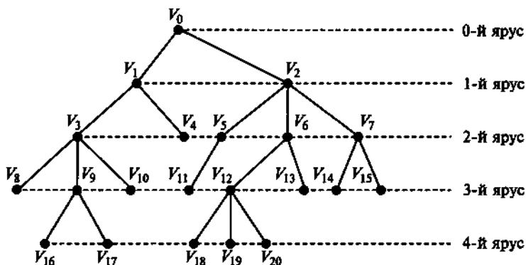
Рис. 2.14. Иллюстрация графа-дерева
