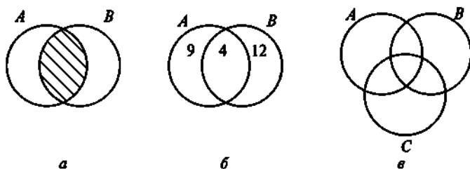
Рис. 1.17. Схемы, иллюстрирующие правило суммы для объединения множеств:
