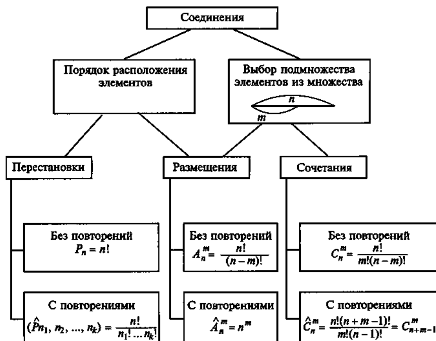
Рис. 1.19. Схема комбинаторных операций
