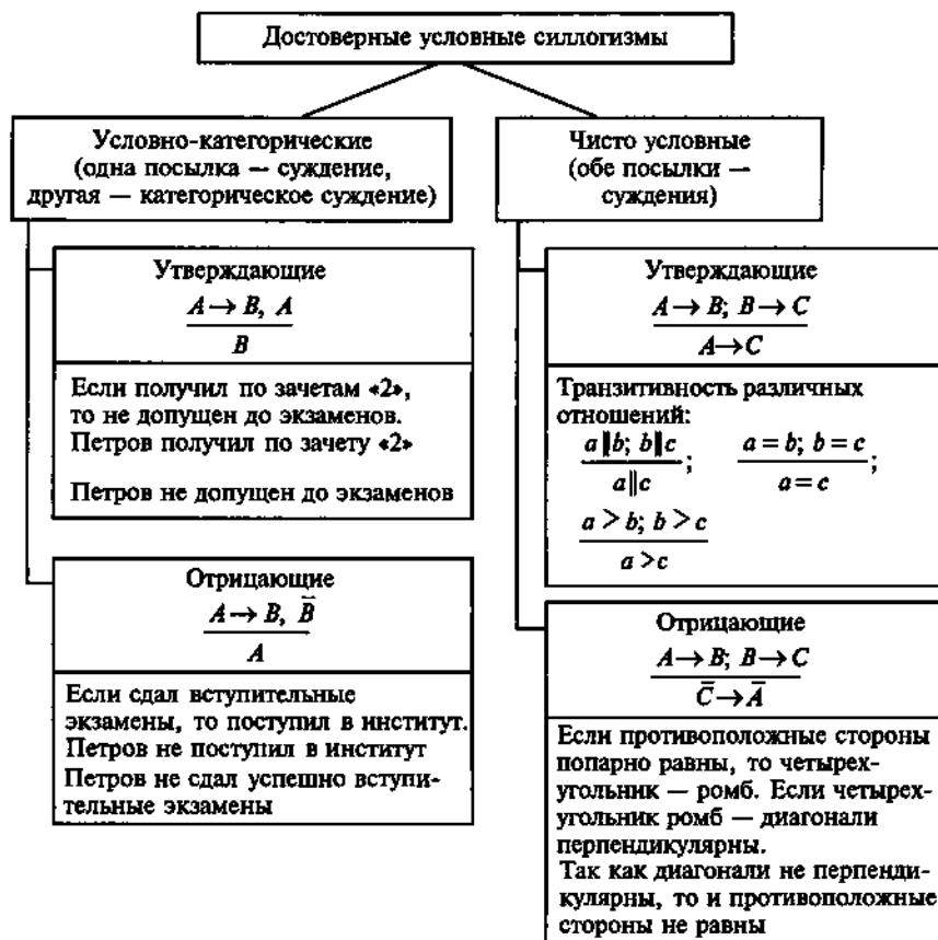
Рис. 5.10. Условные силлогизмы:
