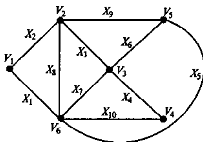
Рис. 2.18. Графическая интерпретация графа G , заданного табл. 2.2
