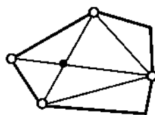
Рис. 1.18. Точки пересечения диагоналей многоугольника
