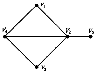
Рис. 2.10. Изображение гамильтоновых путей
