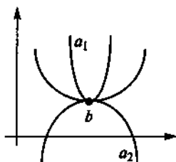
Рис. 1.2. Иллюстрация соответствия R — «вершина параболы»
