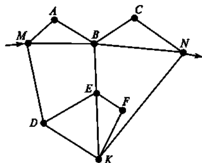
Рис. 2.30. Граф путешествия по историческим местам
