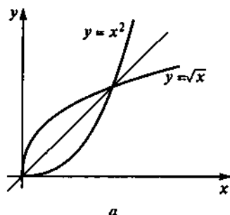
Рис. 1.16. Графики прямых и обратных бинарных отношений:
