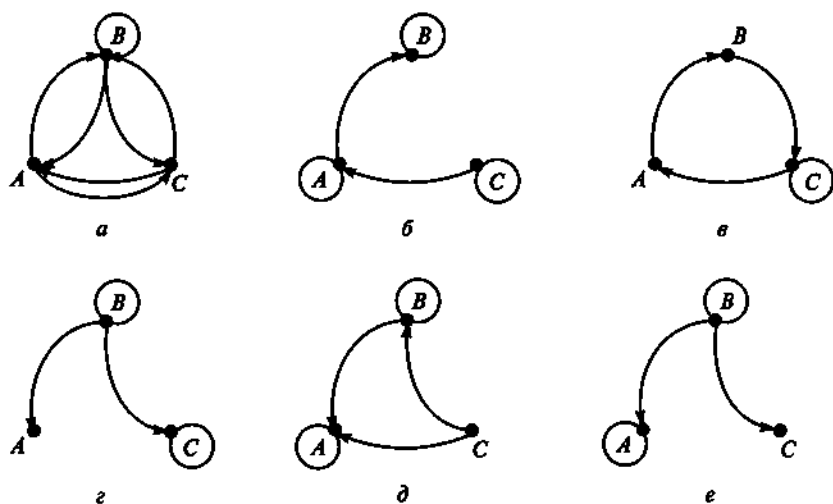
Рис. 2.29. Задание графа G к упр. 2.4 ( a-e — варианты)
