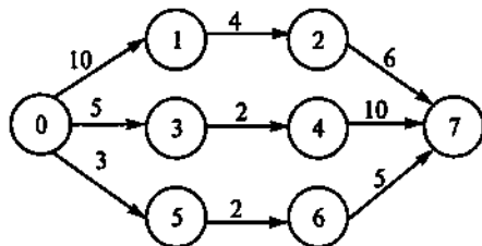
Рис. 2.21. Взвешенный сетевой граф проведения комплекса работ
