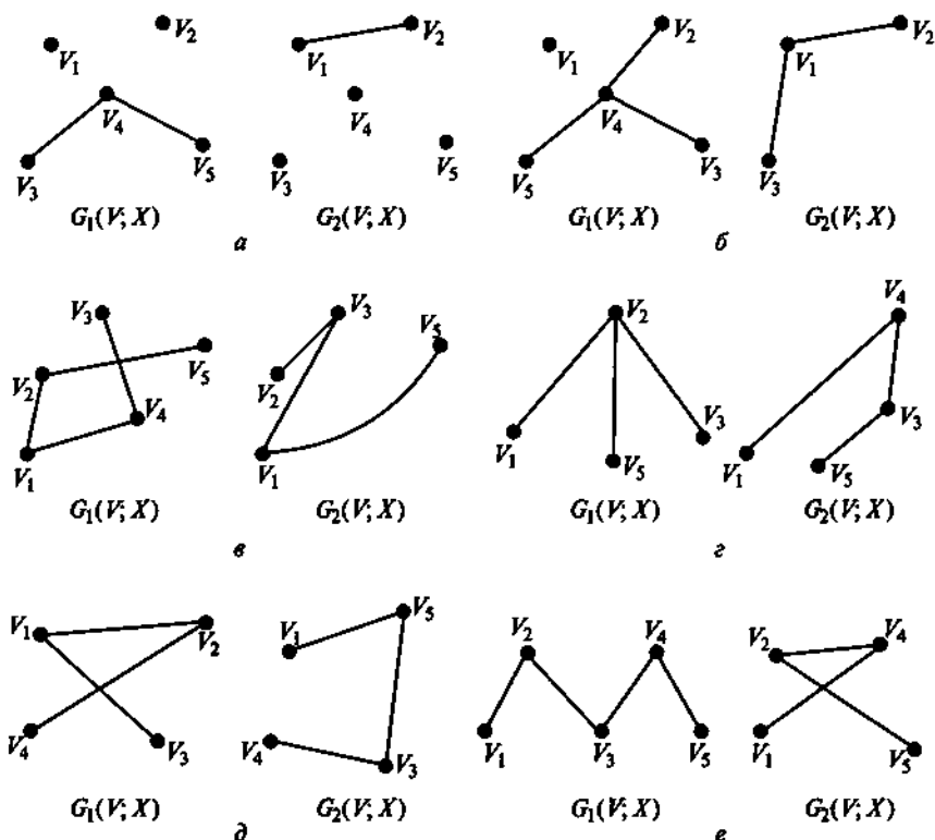
Рис. 2.28. Задание графов G_1 и G_2 к упр. 2.3 ( a-e — варианты)
