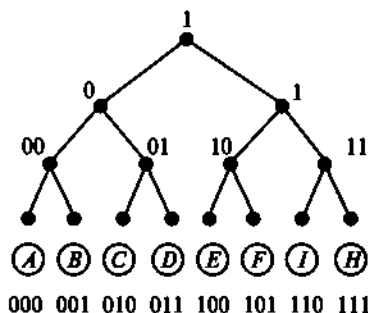
Рис. 6.1. Двоичное дерево для восьми символов
