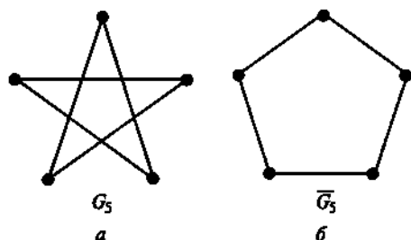
Рис. 2.2. Дополнение \bar{G}_5 графа G_5 до графа G_2 , изображенного на рис. 2.1, б
