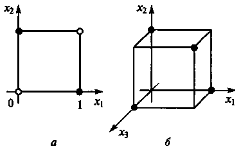
Рис. 4.16. Геометрическая интерпретация суммы по модулю два:
