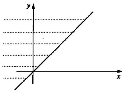
Рис. 1.15. Иллюстрация бинарного отношения R ( x \leq y , где x, y \in \mathbb{R} )
