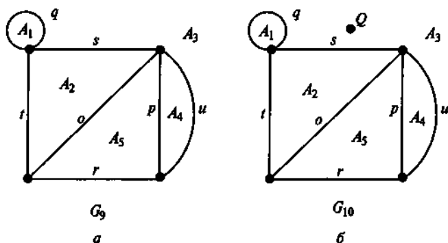
Рис. 2.6. Графы:
