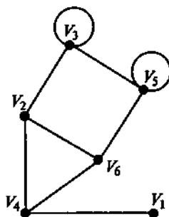
Рис. 2.19. Граф к задаче 20
