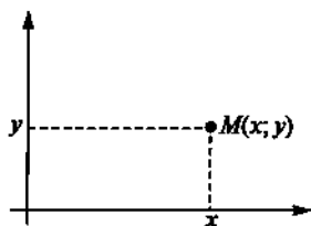
Рис. 1.3. Задание отображения xRy с помощью метода координат
