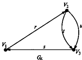
Рис. 2.3. Ориентированный граф
