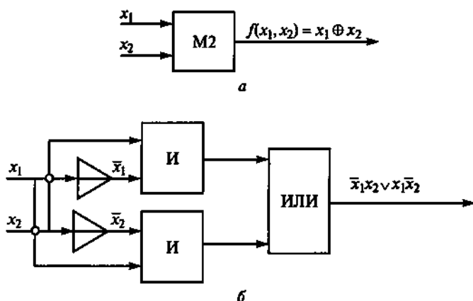
Рис. 4.15. Элемент и схема для операции M2: а — логический элемент; б — логическая схема
