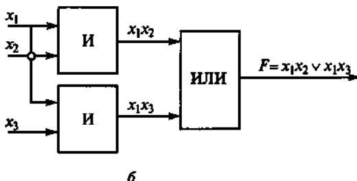
Рис. 4.7. Логическая схема булевой функции F :
