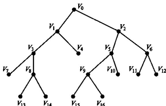
Рис. 2.16. Бинарное дерево
