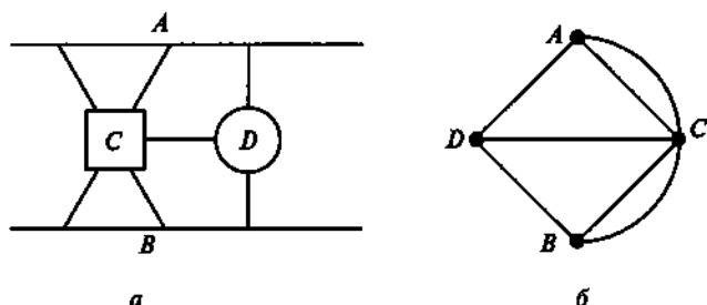
Рис. 2.11. Иллюстрации к задаче «О кёнигсбергских мостах»:
