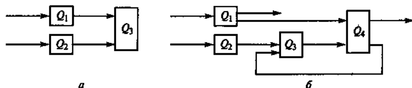
Рис. 7.3. Схема автоматов:
