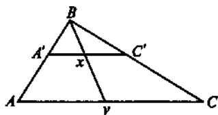
Рис. 1.11. Биекция между средней линией и основанием треугольника
