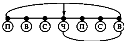
Рис. 6.3. Метод половинного деления
