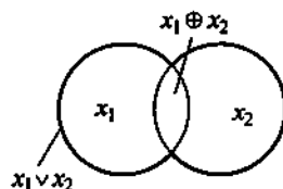
Рис. 4.14. Связь между дизъюнкцией x_1 \vee x_2 и суммой по модулю два
