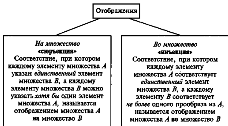
Рис. 1.5. Классификация отображений по мощности
