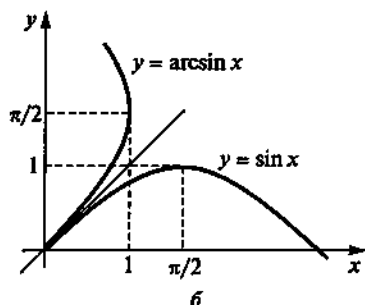
Рис. 1.16. Графики прямых и обратных бинарных отношений:
