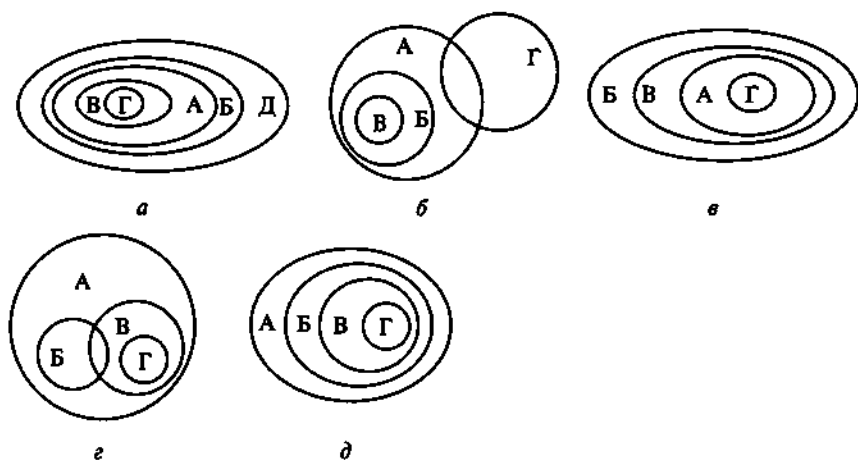
Рис. 3.11. Схемы к упр. 3.8 (а—д — варианты)
