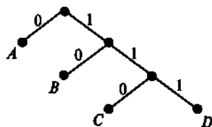
Рис. 6.2. Двоичное дерево для четырех символов
