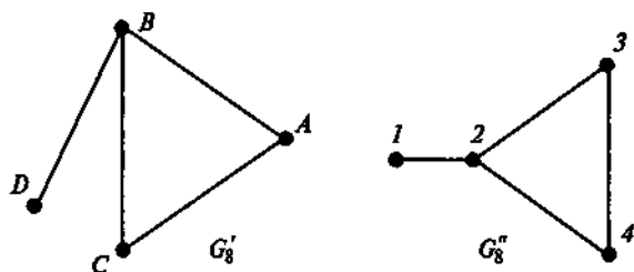
Рис. 2.5. Изоморфные графы
