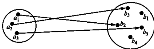
Рис. 1.4. Графическое задание инъективного отображения множества A в B
