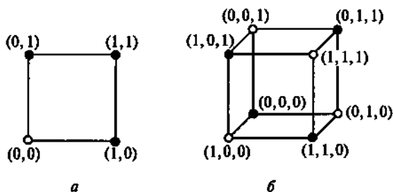
Рис. 4.1. Геометрическая интерпретация булевых функций:
