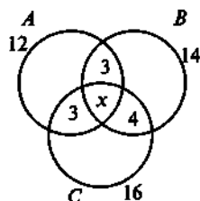
Рис. 1.22. Схематическое изображение условия задачи 16
