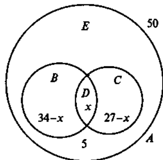
Рис. 1.20. Схематическое изображение условия задачи 14
