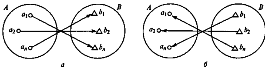
Рис. 1.7. Иллюстрация биекции:
