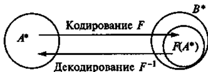
Рис. 6.4. Схема декодирования
