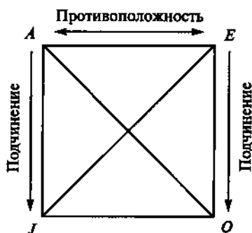
Рис. 5.7. Логический квадрат
