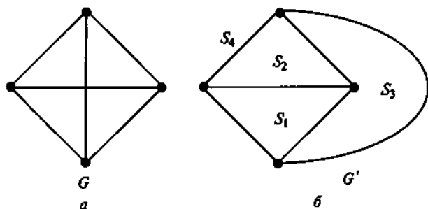
Рис. 2.8. Планарные графы:
