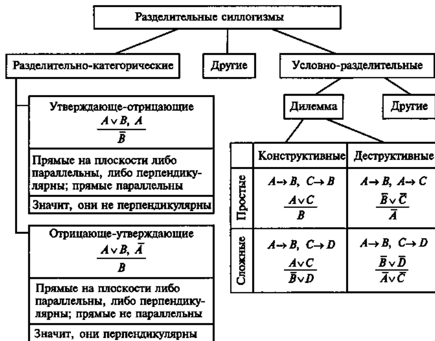
Рис. 5.9. Разделительные силлогизмы
