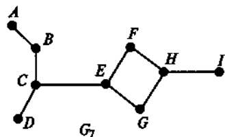
Рис. 2.4. Граф G_7 с мостами BC и CE
