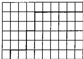
Рис. 1.14. Движение по прямоугольной решетке
