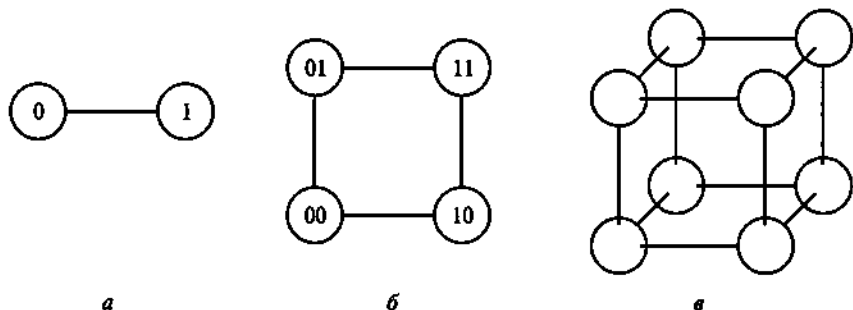
Рис. 1.13. Иллюстрация n -мерного куба:
