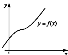
Рис. 1.6. График непрерывного биективного отображения y = f(x)
