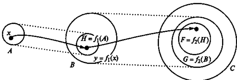
Рис. 1.9. Схема, иллюстрирующая композицию двух инъекций
