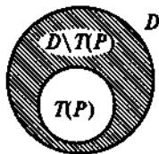
Рис. 5.1. Множество истинности предиката \overline{P(x)}
