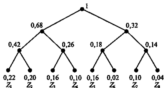
Рис. 6.6. Кодовое дерево для восьми символов с учетом вероятностей
