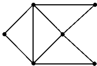
Рис. 2.9. Изображение эйлерова графа
